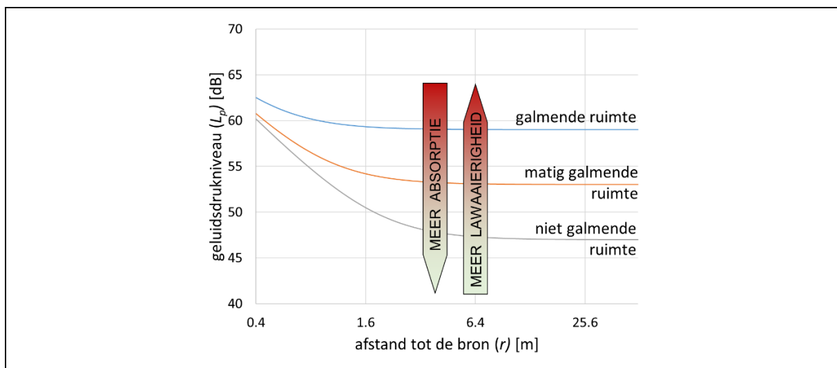
Afb. 4 Verband tussen absorptie en lawaaierigheid in een ruimte.
