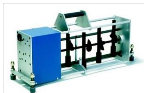
Afb 1. Bepaling van het genormaliseerde contactgeluidsdrukkniveau L_n in het laboratorium volgens NBN EN ISO 10140-3.
