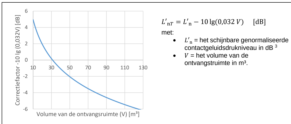
Afb. 3 De geometrische correctiefactor bij contactgeluidsisolatie (in het geval T_0 = 0,5 s en A_0 = 10 m 2 ).
