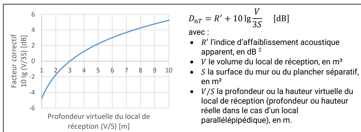
Fig. 3 Facteur de correction géométrique applicable à l'isolement au bruit aérien (si T_0 = 0,5 s).
