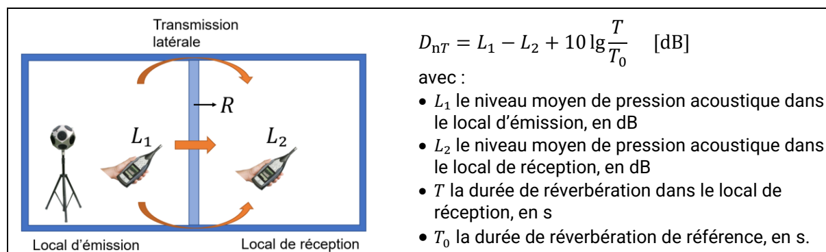
Fig. 2 Détermination in situ de l'isolement acoustique standardisé D_{nT} entre deux locaux selon la norme NBN EN ISO 16283-1.
