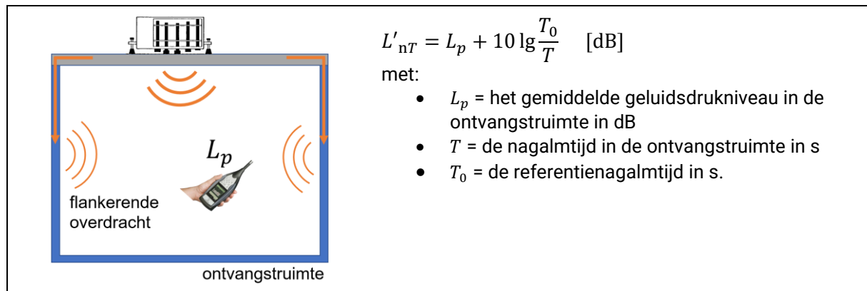
Afb. 2 Bepaling van het gestandaardiseerde contactgeluidsdrukkniveau L'_{nT} in situ volgens NBN EN ISO 16283-2
