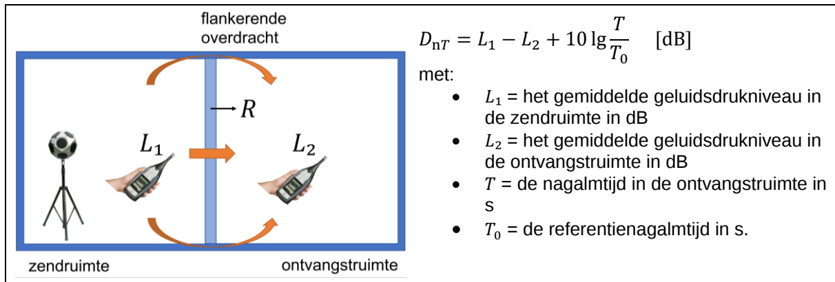
Afb. 2 Bepaling van het gestandaardiseerde geluidsdruk-niveauverschil D_{nT} tussen twee kamers in situ volgens NBN EN ISO 16283-1.
