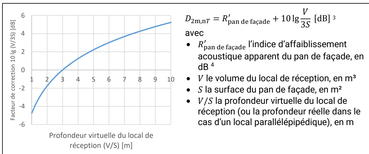
Figure 5 Facteur de correction géométrique applicable à l'isolement d'un pan de façade (si T_0 = 0,5 s).
