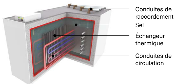
1 Coupe et composants internes de la batterie PCM testée.
