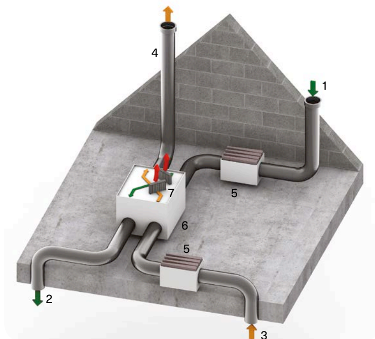
3 Schéma de l'utilisation des filtres à poches dans une ventilation résidentielle double flux.
