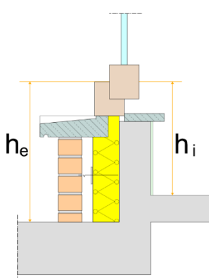
Afbeelding 12 De referentiehoogtes h_i en h_e voor de beschermingshoogte H .
