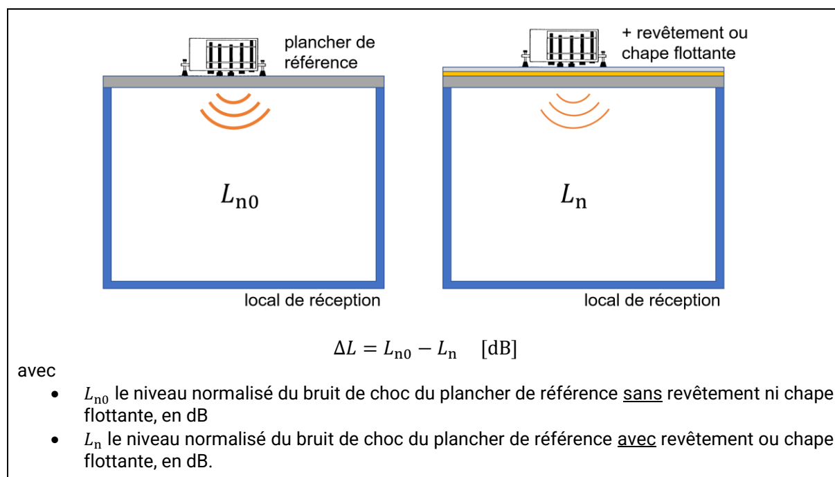
Figure 4 Détermination en laboratoire de la réduction du niveau du bruit de choc \Delta L selon l'Annexe H de la norme NBN EN ISO 10140-1.
