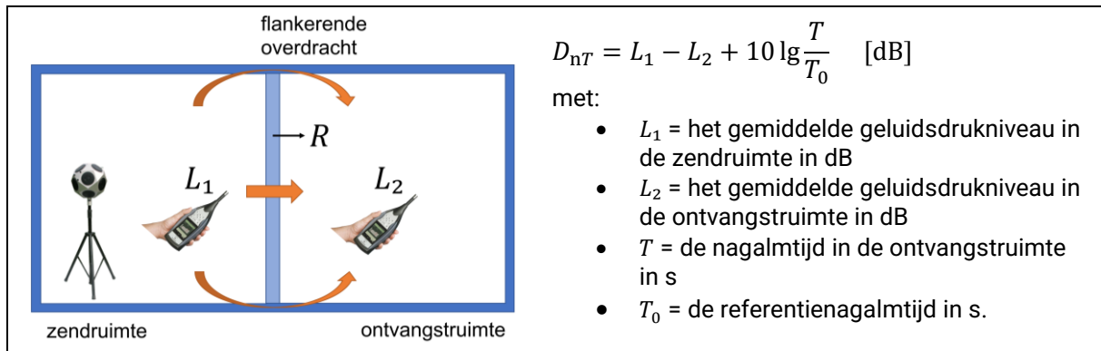
Afb. 2 Bepaling van het gestandaardiseerde geluidsdruk-niveauverschil D_{nT} tussen twee kamers in situ volgens NBN EN ISO 16283-1.
