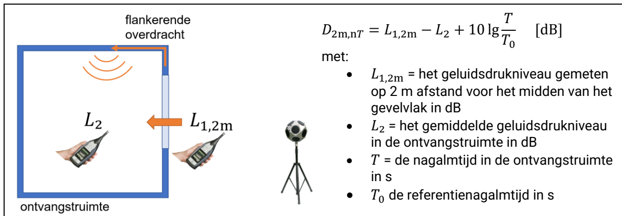
Afb. 4 Bepaling van het gestandaardiseerde geluidsdruk niveauverschil D_{2m,nT} van een gevelvlak in situ volgens NBN EN ISO 16283-3
