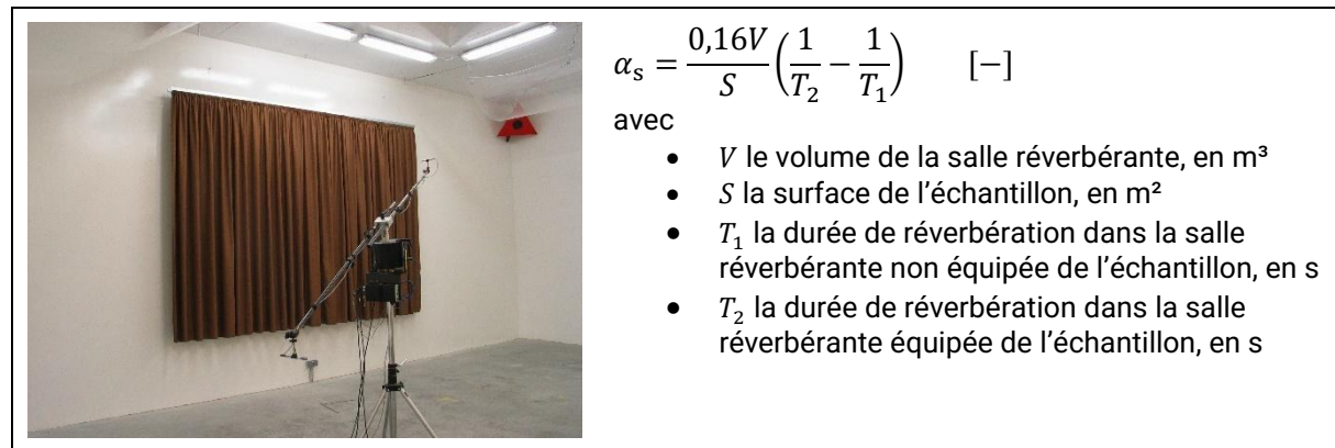
Figure 2 Détermination du coefficient d'absorption \alpha_s sous incidence diffuse du bruit en salle réverbérante selon la norme NBN EN ISO 354.
