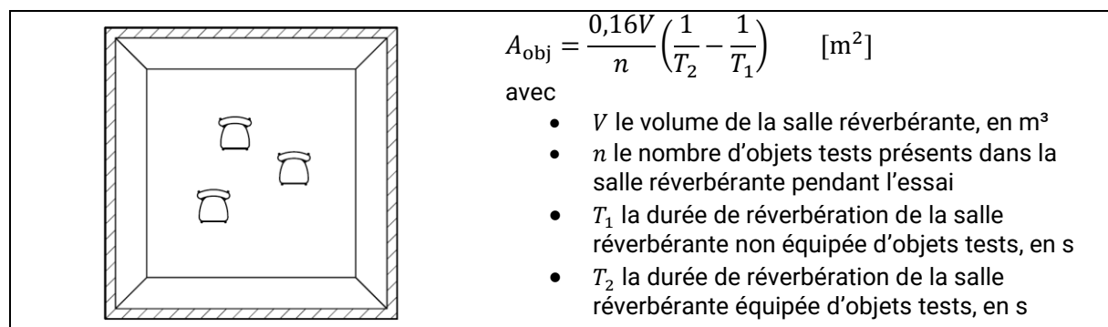
Figure 3 Aire d'absorption équivalente A_{\text{obj}} d'un objet déterminée en laboratoire selon NBN EN ISO 354.
