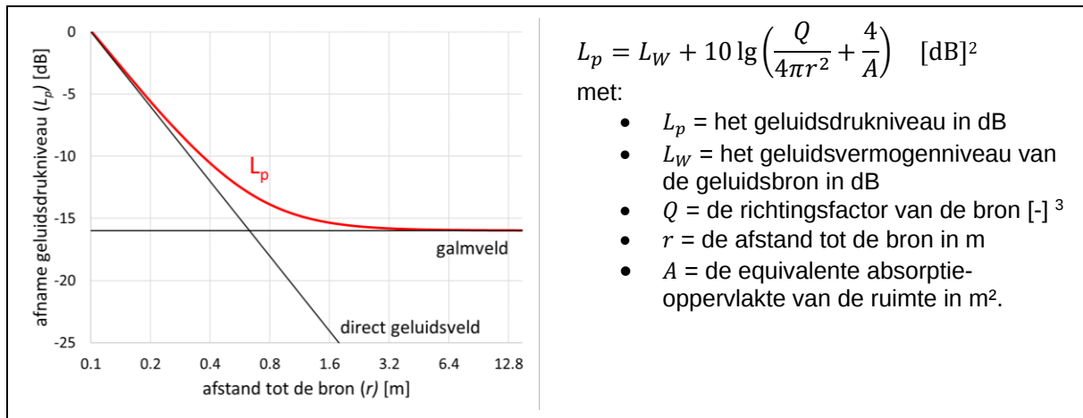
Afb. 3 Direct geluidsveld en galmveld in een ruimte.
