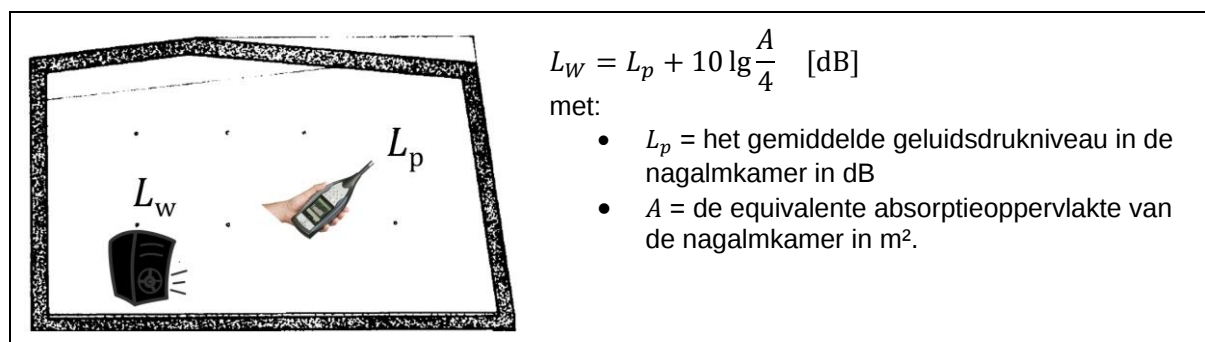
Afb. 1 Bepaling van het geluidsvermogeniveau L_W in het laboratorium volgens de nagalmkamer methode uit NBN EN ISO 3741.
