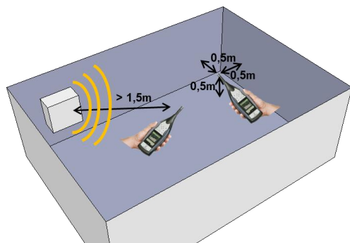
Afb. 2 Bepaling van het gemiddelde geluidsdruk niveau in een ruimte volgens NBN EN ISO 16032 of NBN EN ISO 10052
