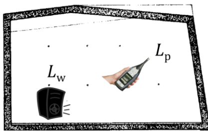
Afb. 1 Bepaling van het geluidsvermogeniveau L_W in het laboratorium volgens de nagalmkamer methode uit NBN EN ISO 3741.
