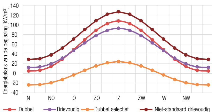
1 | Balans van de warmteverliezen en de zonnewinsten in de winter, doorheen 1 m 2 beglazing met een helling van 45°
