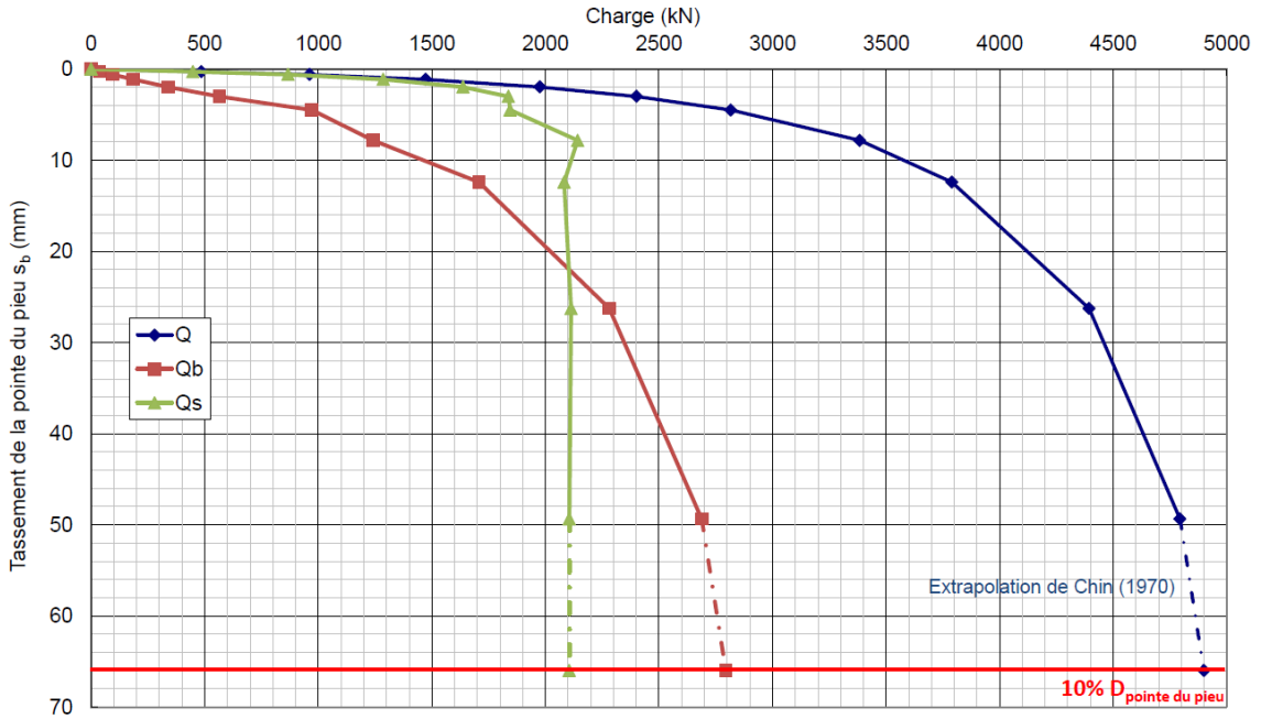
Essai de chargement statique - Haren - Franki - 5.12.2013
