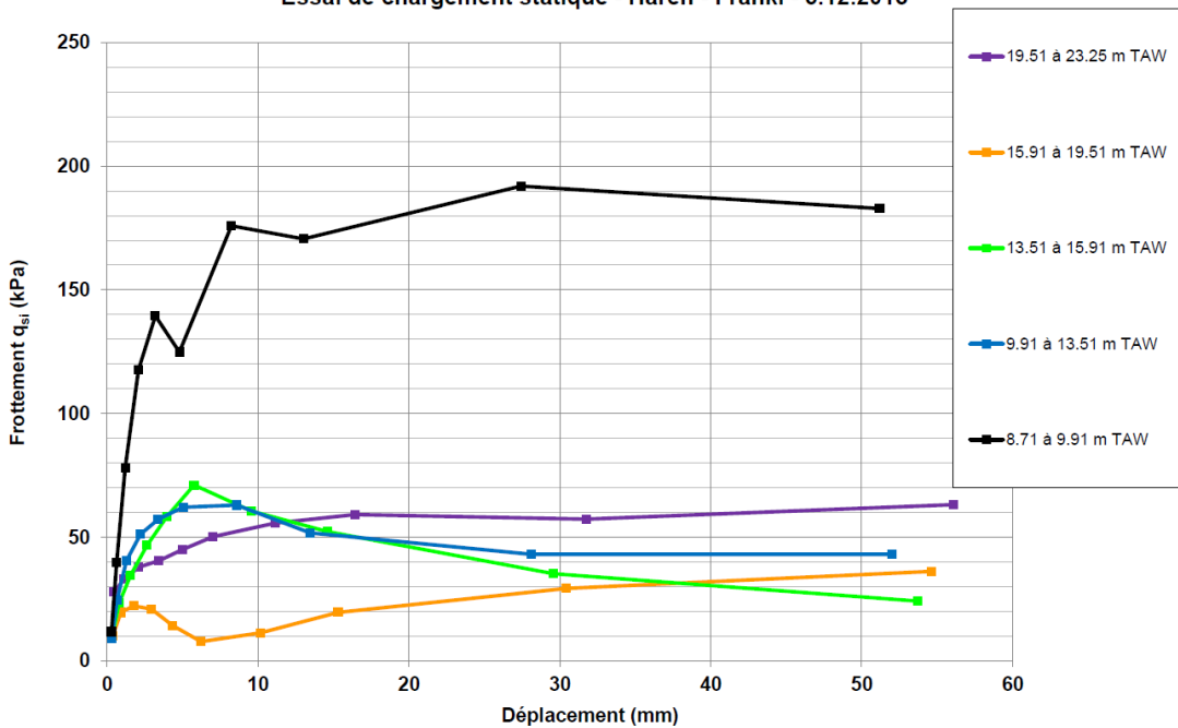
Essai de chargement statique - Haren - Franki - 5.12.2013
