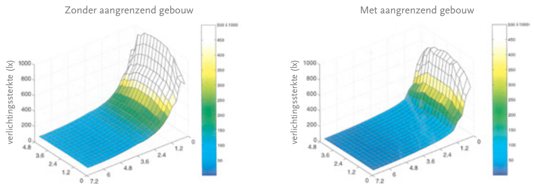
▲ Impact van een stedelijke obstructie op de verlichtingssterkte in een lokaal Bron: onderzoeksgroep Architecture et Climat van Université Catholique de Louvain (UCL)
